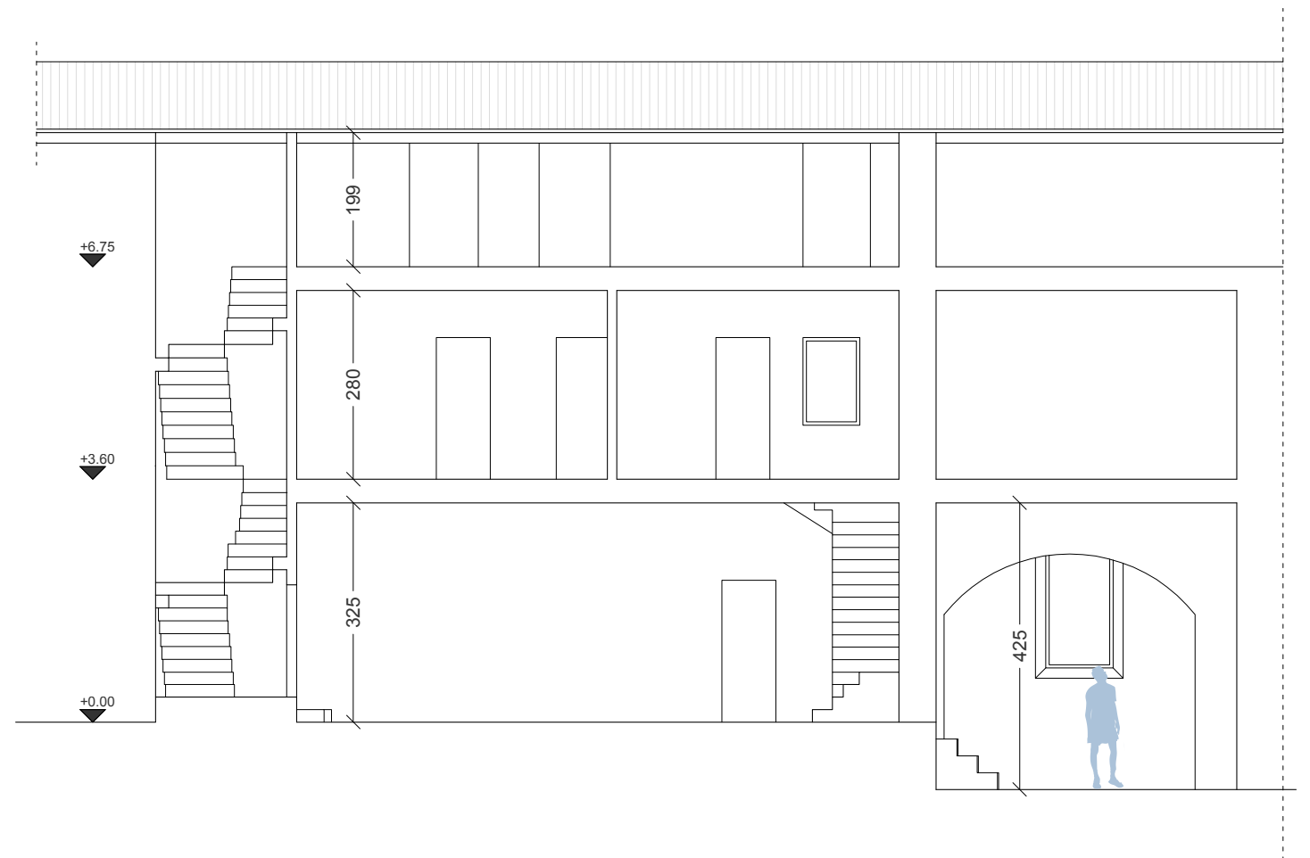
sezione BB
